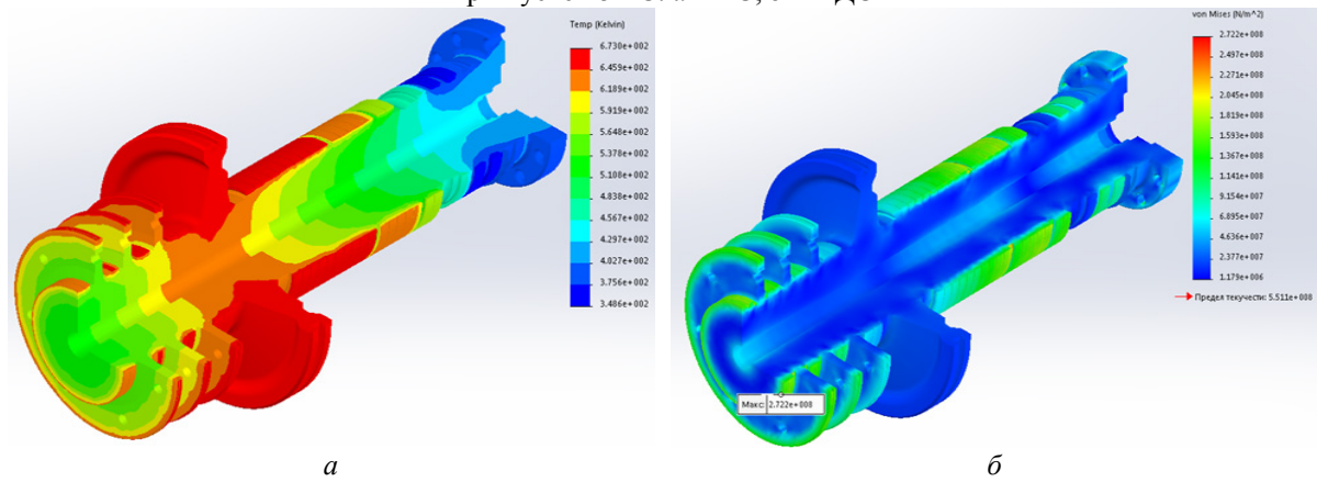
Рис. 2 – Результаты оценки ротора ВД в момент времени 1900 с (нагрузка до 30 МВт) при пуске из ХС-2: а – ТС; б – НДС
