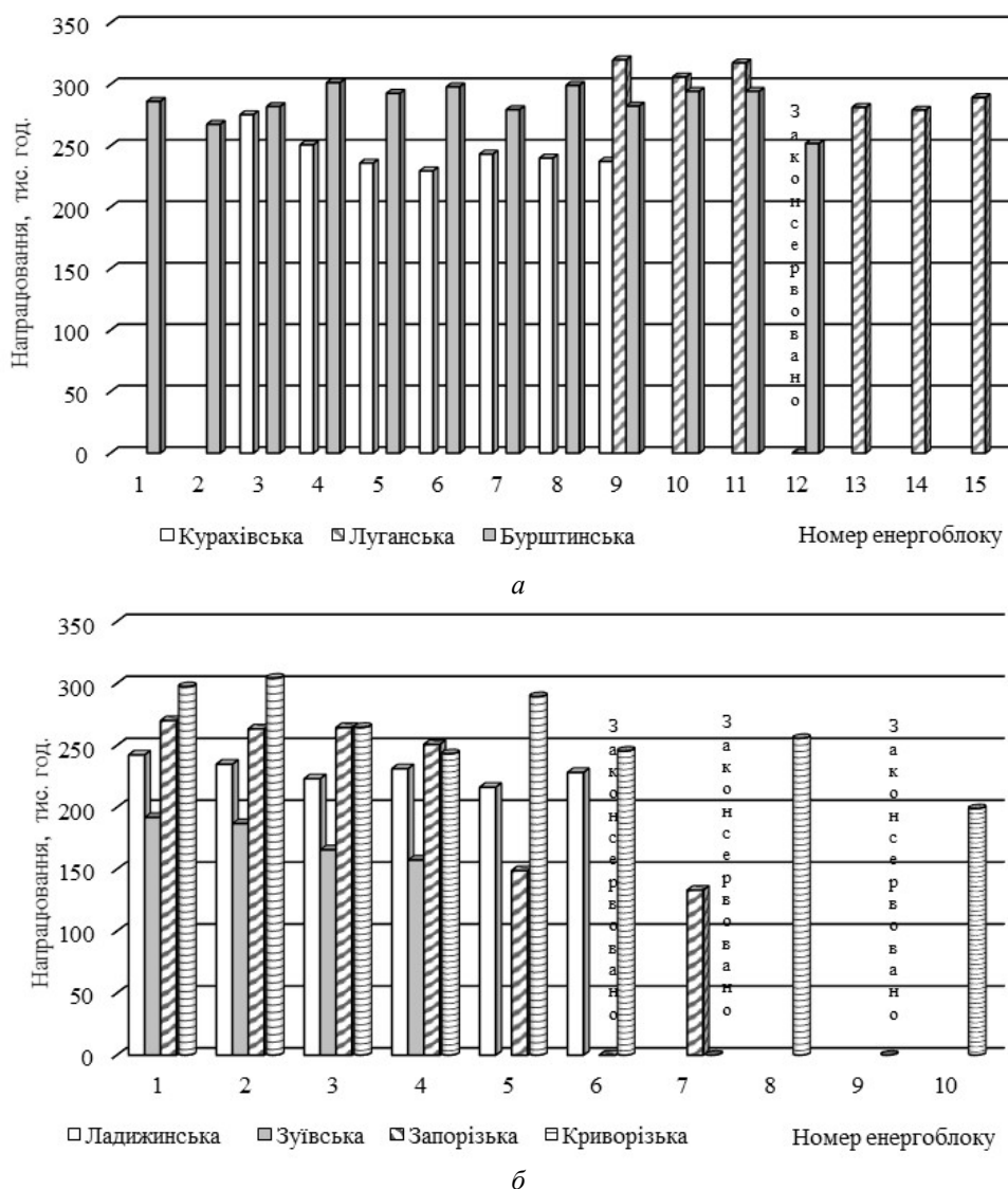
Рис. 1 – Напрацювання турбін теплових електростанцій ДТЕК станом на 01.01.2015 р.: а – напрацювання турбін потужністю 200 МВт; б – напрацювання турбін потужністю 300 МВт
