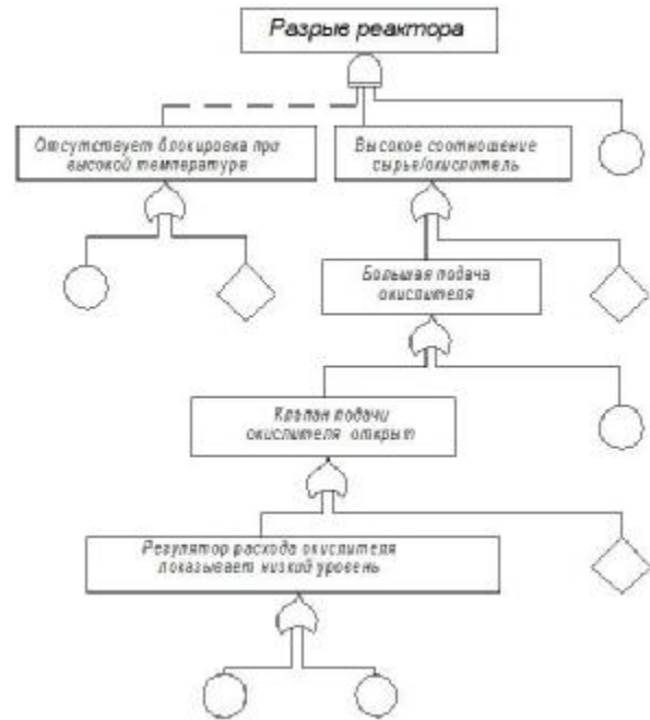
Рис. 7 – «Дерево отказов» для описания возникновения аварий в реакторах энергоблоков АЭС
