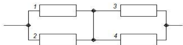
Рис. 4 – Мостиковая схема соединений при безусловно исправном элементе «5» схемы на рис. 1
