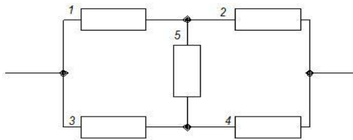
Рис. 1 – Мостиковая схема участка технологической системы подвода питательной воды к парогенераторам АЭС: элементы «1», «2», «3», «4» – отдельные участки трубопроводов с арматурой; элемент «5» – перемычка между ними
