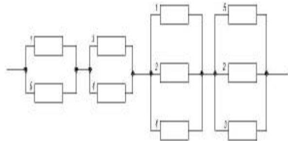
Рис. 3 – Минимальные сечения для мостиковой схемы на рис. 1
