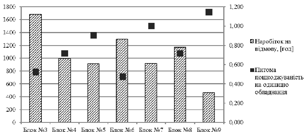
Рис. 1 – Діаграма розподілення наробітку на відмову та питомої пошкоджуваності на одиницю обладнання для КуТЕС
