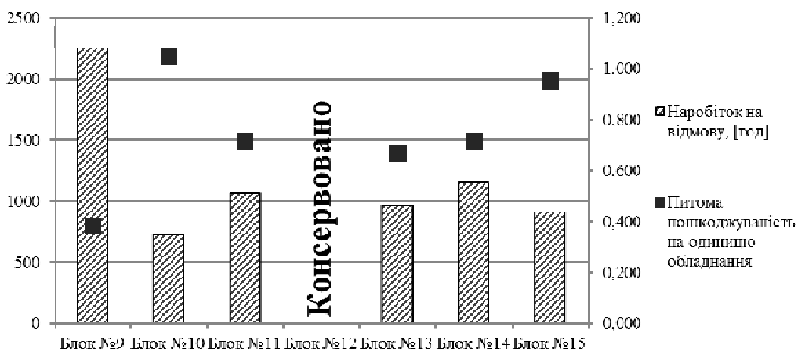
Рис. 2 – Діаграма розподілення наробітку на відмову та питомої пошкоджуваності на одиницю обладнання для ЛуТЕС
