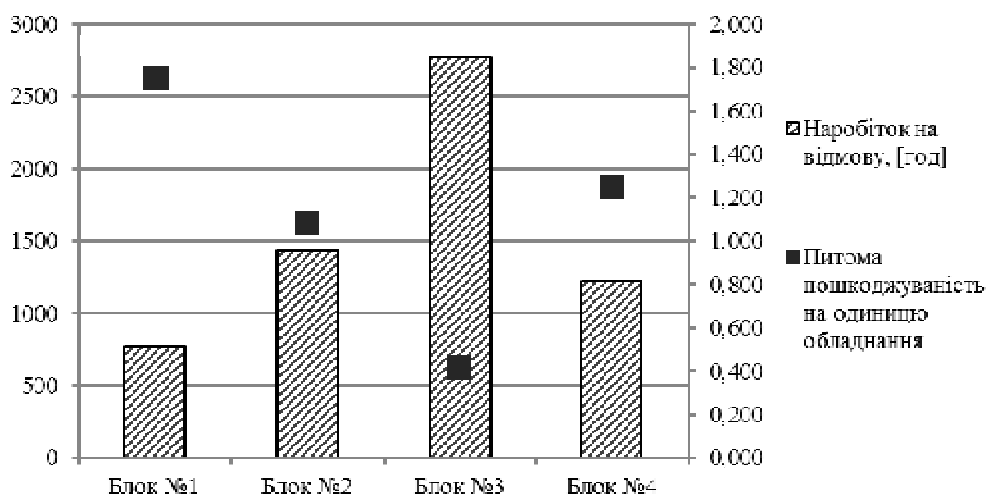
Рис. 3 – Діаграма розподілення наробітку на відмову та питомої пошкоджуваності на одиницю обладнання для ЗаТЕС
