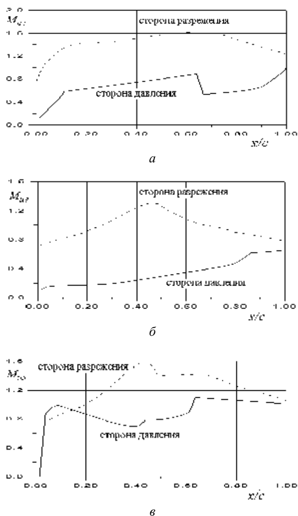
Рис. 6 – Мгновенное распределение скорости по обводу профиля рабочей лопатки: а – периферийное сечение; б – среднее сечение; в – корневое сечение
