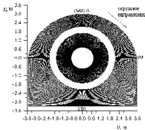
Рис. 2 – Разностная сетка для выхлопного патрубков в плоскости перпендикулярной оси вращения (плоскости x-y )
