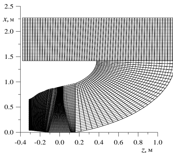
Рис. 1 – Разностная сетка для статора, ротора и выхлопного патрубков в меридиональной плоскости (плоскости x-z )
