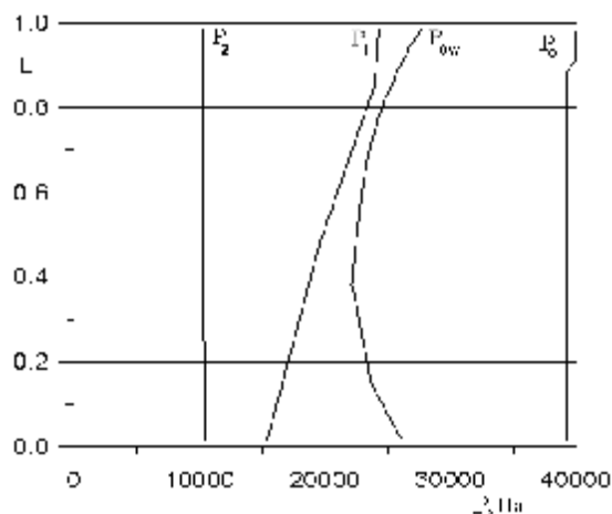
Рис. 4 – Распределение давления по высоте лопатки
