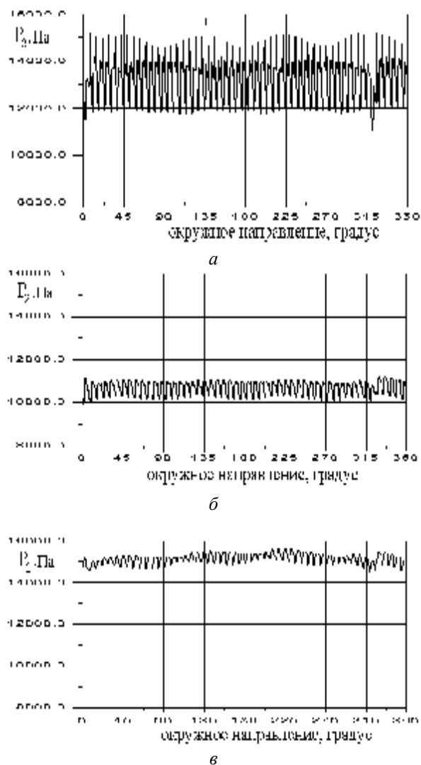
Рис. 5 – Распределение статического давления в окружном направлении за ротором: а – периферийное сечение; б – среднее сечение; в – корневое сечение
