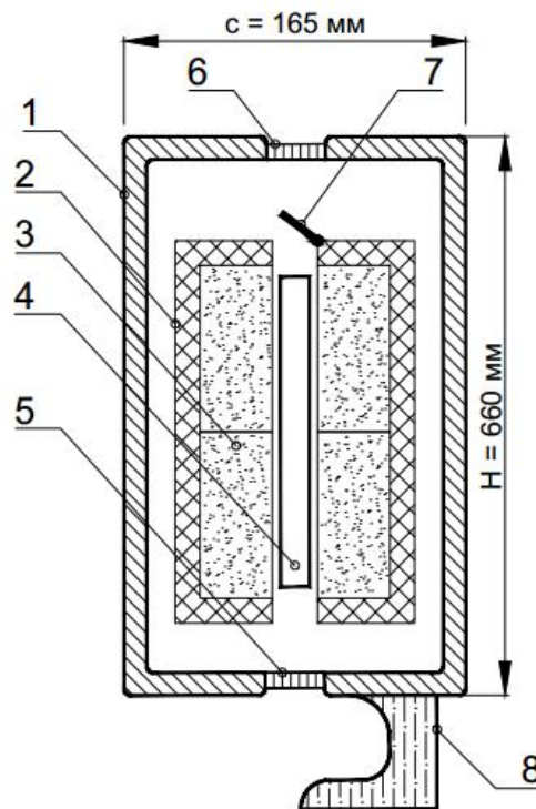
Рис. 1 – Принципова схема статичного ТАЕП [4]: 1 – зовнішня оболонка (кожух); 2 – теплоізоляційний прошарок; 3 – теплоакumuлюючий матеріал; 4 – електричний нагрівач; 5 – решітка для входу повітря; 6 – решітка для виходу повітря; 7 – регулюючий клапан; 8 – підставка
