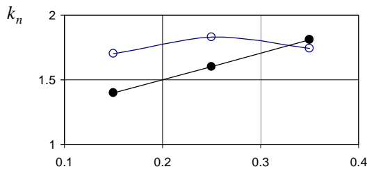
● – \bar{S} = 0,114 ; ○ – \bar{S} = 0,3 G_{\text{отб}}
