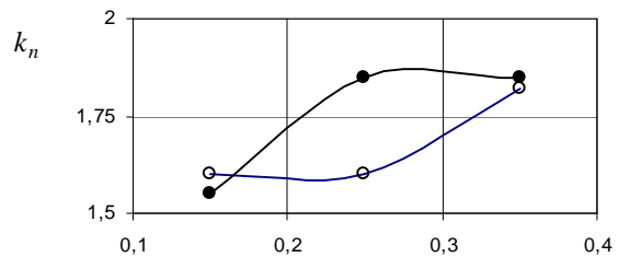
● – \bar{S} = 0,106 ; ○ – \bar{S} = 0,343 G_{\text{отб}}
