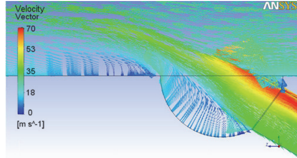
Рис. 5 – Структура потока в полусферическом углублении ( m = 1,5 )
