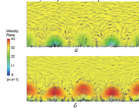
Рис. 7 – Векторы скорости при x/d = 3 за вторым рядом отверстий; m = 1,5 : а – отверстия в полусферических углублениях; б – цилиндрические отверстия в стенке
